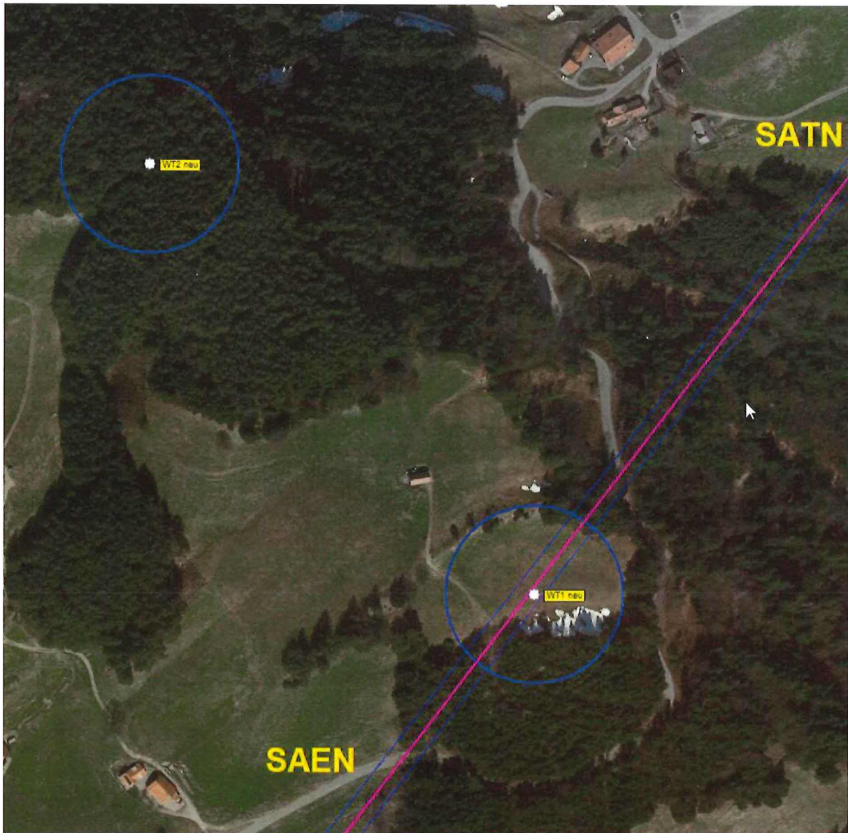
Abbildung 48: Störung des Richtfunks der SRG Sântis-St.Anton
