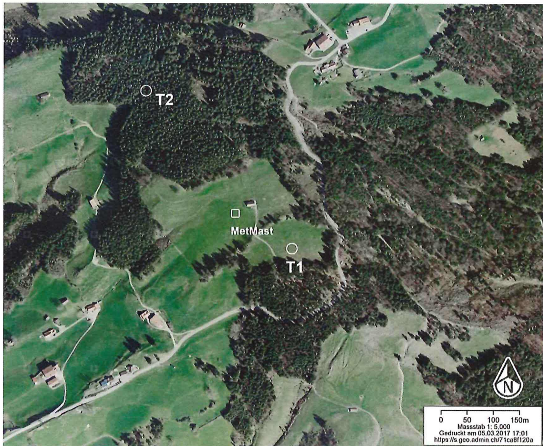
Abbildung 11: Vorgesehene Anlagenpositionen T1 und T2, sowie Position des Windmessmastes
